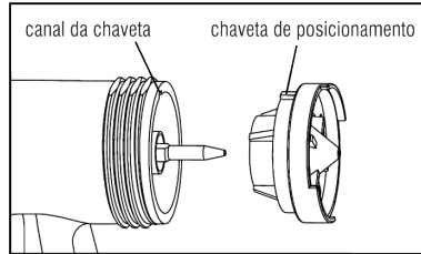
Fig. 9 - Montagem da capa de ar
