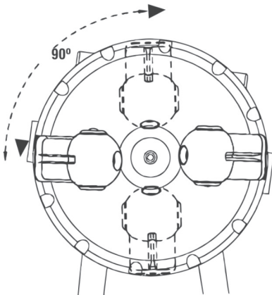
Fig. 4 - Ajustando el chorro de pintura
